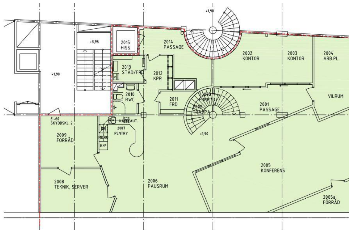
Källarplan
